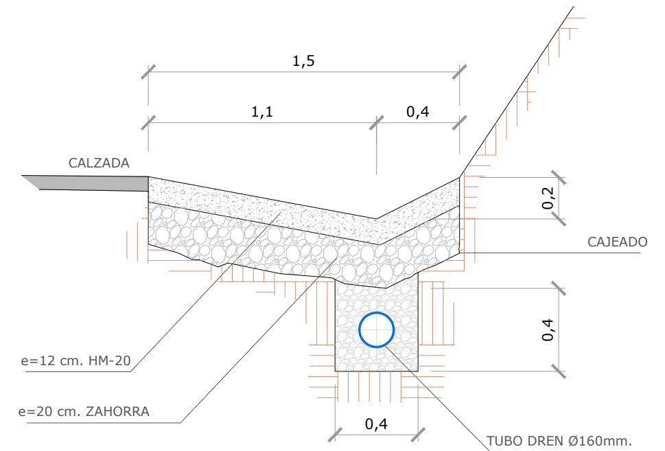
CUNETA TIPO 2. REBASABLE ESCALA 1:25
