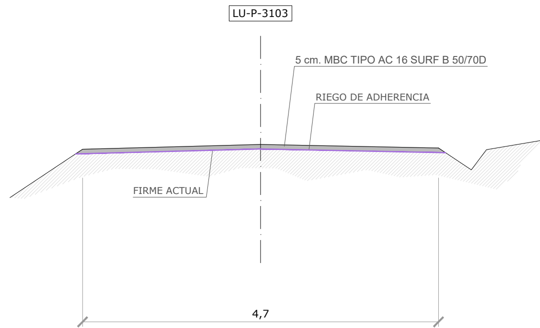
SECCIÓN TIPO. LU-P-3103 ESCALA 1:50
