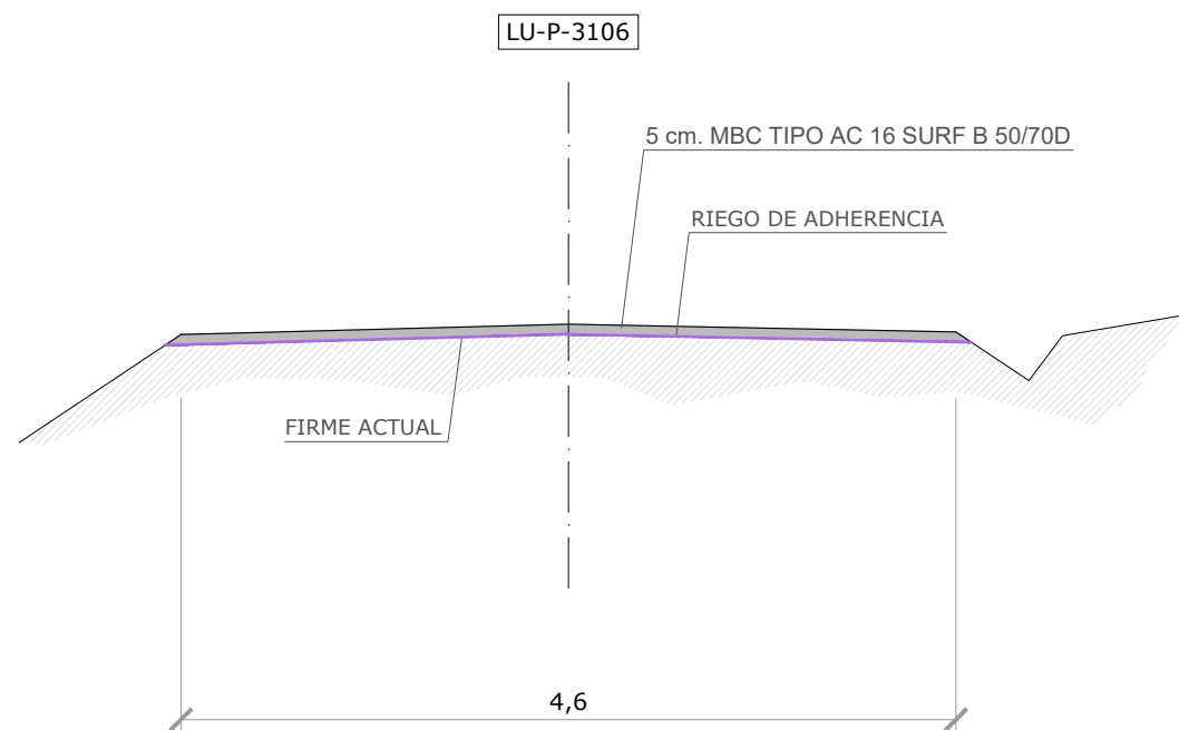
SECCIÓN TIPO. LU-P-3106 ESCALA 1:50
